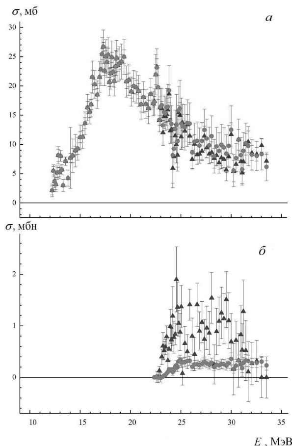
Рис. 3. Сравнение оцененных ([23] — кружки) и экспериментальных ([27] — треугольники) сечений парциальных фотонейтронных реакций для ядра ^{58}\text{Ni} : а — \sigma(\gamma, 1n) , б — \sigma(\gamma, 2n)
