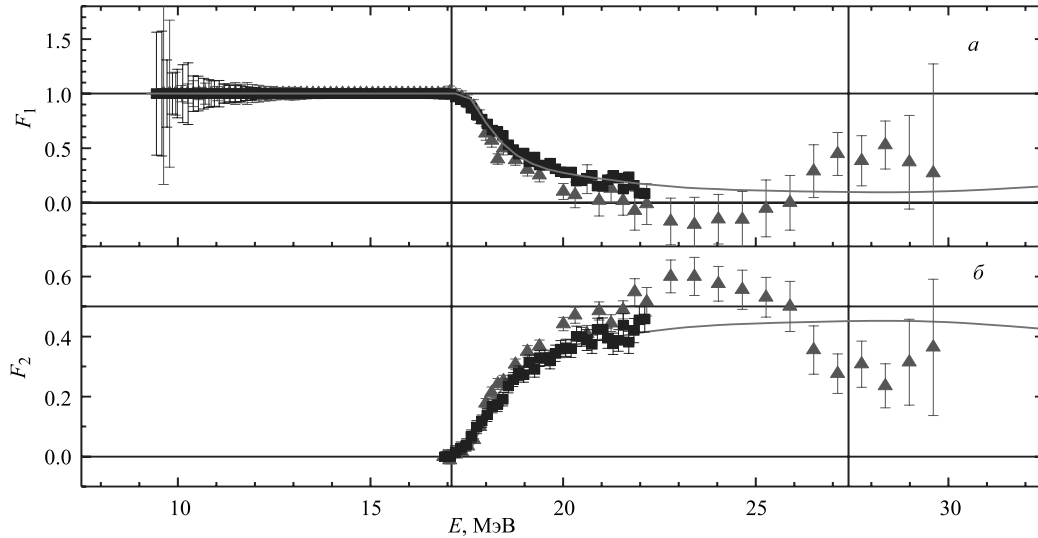
Рис. 2. Отношения F_1^{\text{эксп}} (а) и F_2^{\text{эксп}} (б) для ядра ^{116}\text{Sn} (Ливермор [12] — треугольники и Сакле [13] — квадраты) и F_{1,2}^{\text{теор}} (линии — результаты расчётов в рамках КМФЯР [14, 15])
