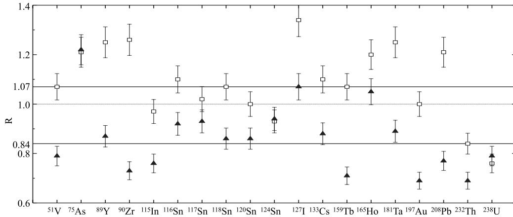
Рис. 1. Полная систематика отношений R интегральных сечений парциальных реакций и полученных в Ливерморе и Сакле [9]: квадраты — данные для реакции (\gamma, 1n) , треугольники — (\gamma, 2n)
