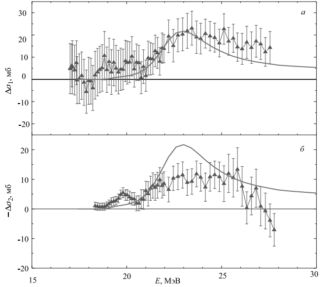
Рис. 4. Сравнение разностей между экспериментальными [28] — треугольники и оцененными [22] сечениями реакций ^{59}\text{Co}(\gamma, 1n)^{58}\text{Co} ( \Delta\sigma_1 ) и ^{59}\text{Co}(\gamma, 2n)^{57}\text{Co} ( \Delta\sigma_2 ) с сечением реакции ^{59}\text{Co}(\gamma, 1n1p)^{57}\text{Fe} , рассчитанным в КМФЯР [14, 15]
