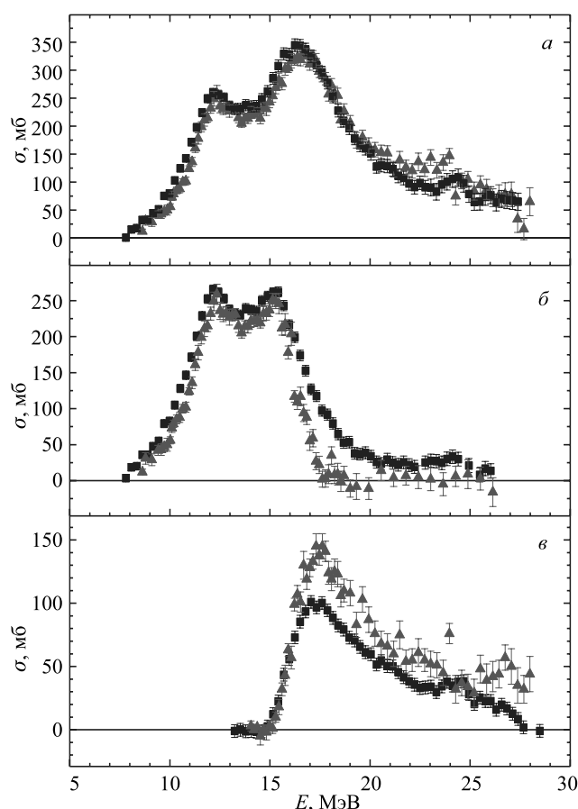
Рис. 5. Сравнение экспериментальных ([29] — треугольники, [30] — квадраты) сечений полных и парциальных реакций на ядре ^{159}\text{Tb} : а — (\gamma, xn) , б — (\gamma, 1n) , в — (\gamma, 2n)
