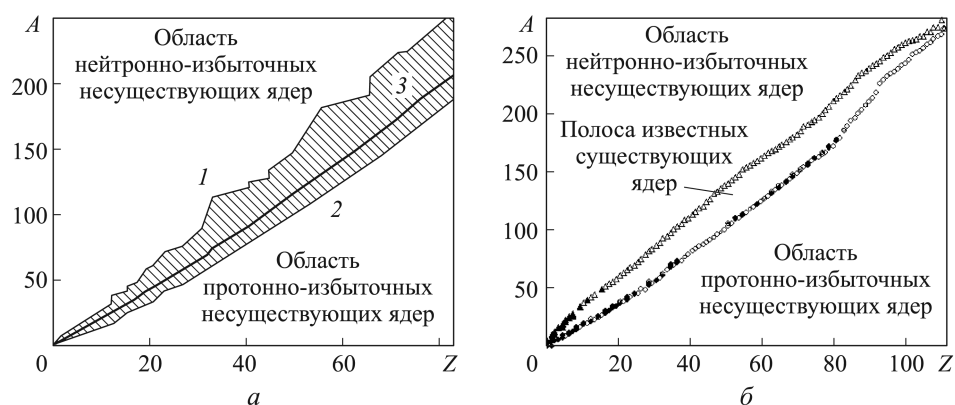
Рис. 1. Области существующих (а) и известных (б) ядер:
