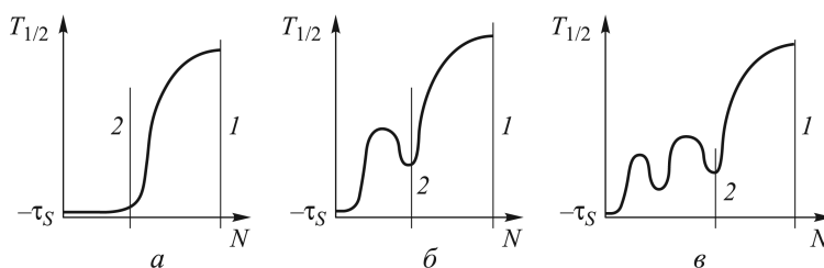
Рис. 4. Зависимости T_{1/2}(N) для протонно-избыточных нуклидов без учета эффектов спаривания и магичности:
