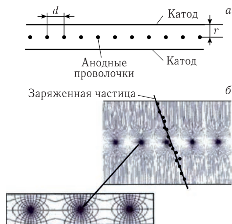
Рис. 8.12. Схема многопроволочной пропорциональной камеры (а) и распределение потенциалов внутри камеры (б). Типичные параметры: d = 1 мм, r = 5\text{--}8 мм, диаметр проволочки — 20 мкм
