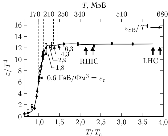
Рис. 10.3. Зависимость плотности энергии КГП из трех ароматов в расчетах КХД на решетках от T/T_c . Критическая температура T_c = 170 МэВ. Вертикальными стрелками указаны температуры, достигнутые на коллайдерах RHIC и LHC. Справа вверху показано предельное значение плотности энергии для идеального газа невзаимодействующих кварков и глюонов
