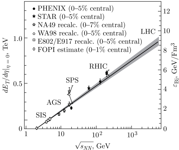
Рис. 4.5. Измеренная поперечная энергия на единицу быстроты при \eta = 0 и бьёркеновская плотность энергии рожденного сгустка материи при \tau_0 = 1 Фм/с (правая шкала) в центральных столкновениях тяжелых ионов
