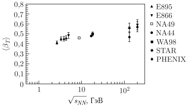
Рис. 10.11. Зависимость средней скорости расширения файерболла от энергии столкновения
