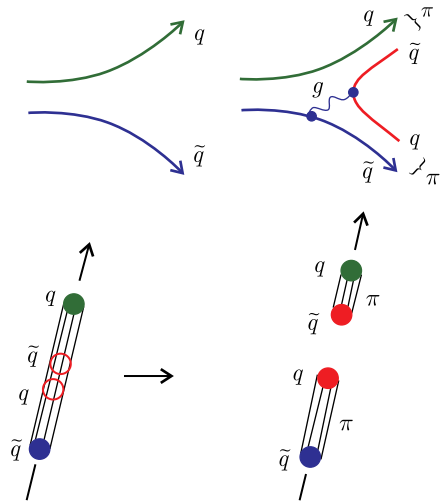
Рис. 1.8. Аналогия проявления не убывающих с расстоянием хромодинамических сил между цветными кварками
