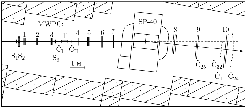
Рис. 9.42. Схема установки ANOMALON: MWPC 1–10 — многопроволочные пропорциональные камеры; S_1 – S_3 — сцинтилляционные счетчики; \check{C}_I , \check{C}_{II} , \check{C}_I – \check{C}_{32} — черенковские счетчики; Т — жидководородная мишень; SP-40 — анализирующий магнит
