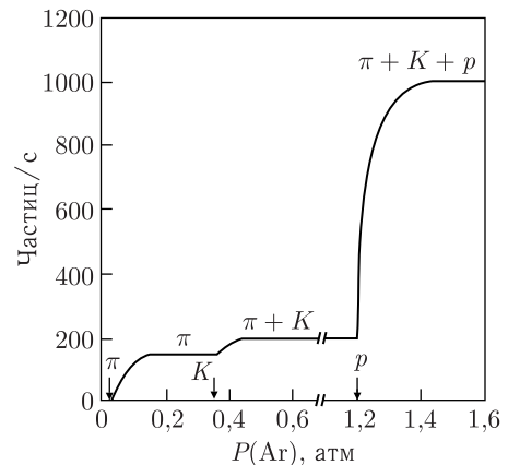
Рис. 8.7. Зависимость скорости счета частиц в пучке с импульсом 35 ГэВ/с от давления аргона в пороговом черенковском счетчике. Стрелками показаны пороги
