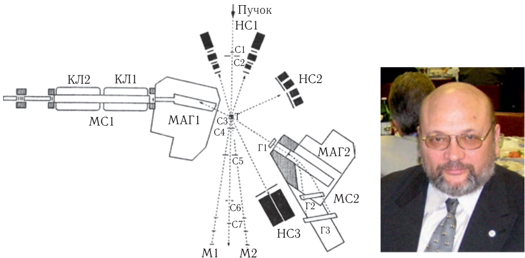
Рис. 9.5. Слева: схема установки «Диск»: МС1, МС2 — магнитные спектрометры; МАГ1, МАГ2 — отклоняющие магниты; КЛ1, КЛ2 — квадрупольные магнитные линзы; Г1–Г3 — годоскопические счетчики; С1 — пучковый счетчик; С2 — вето-счетчик; Т — мишень; С3 — счетчик взаимодействия; С4, С5 — счетчики множественности; С6 — счетчик малых углов; С7 — счетчик фрагментов; М1, М2 — левый и правый мониторы; НС1–НС3 — немагнитные спектрометры. Справа: Ю. А. Панебратцев — руководитель работ на установке «Диск»
