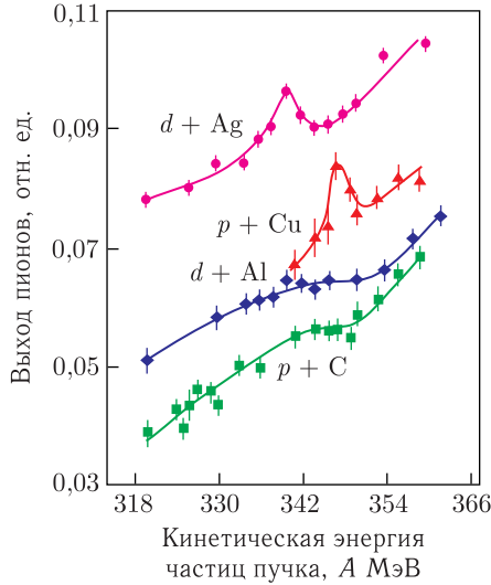
Рис. 9.35. Выход пионов в результате взаимодействия дейтронов и протонов с различными ядрами в зависимости от энергии налетающих частиц. Хорошо виден повышенный выход пионов в области энергии частиц пучка 335–355 А МэВ
