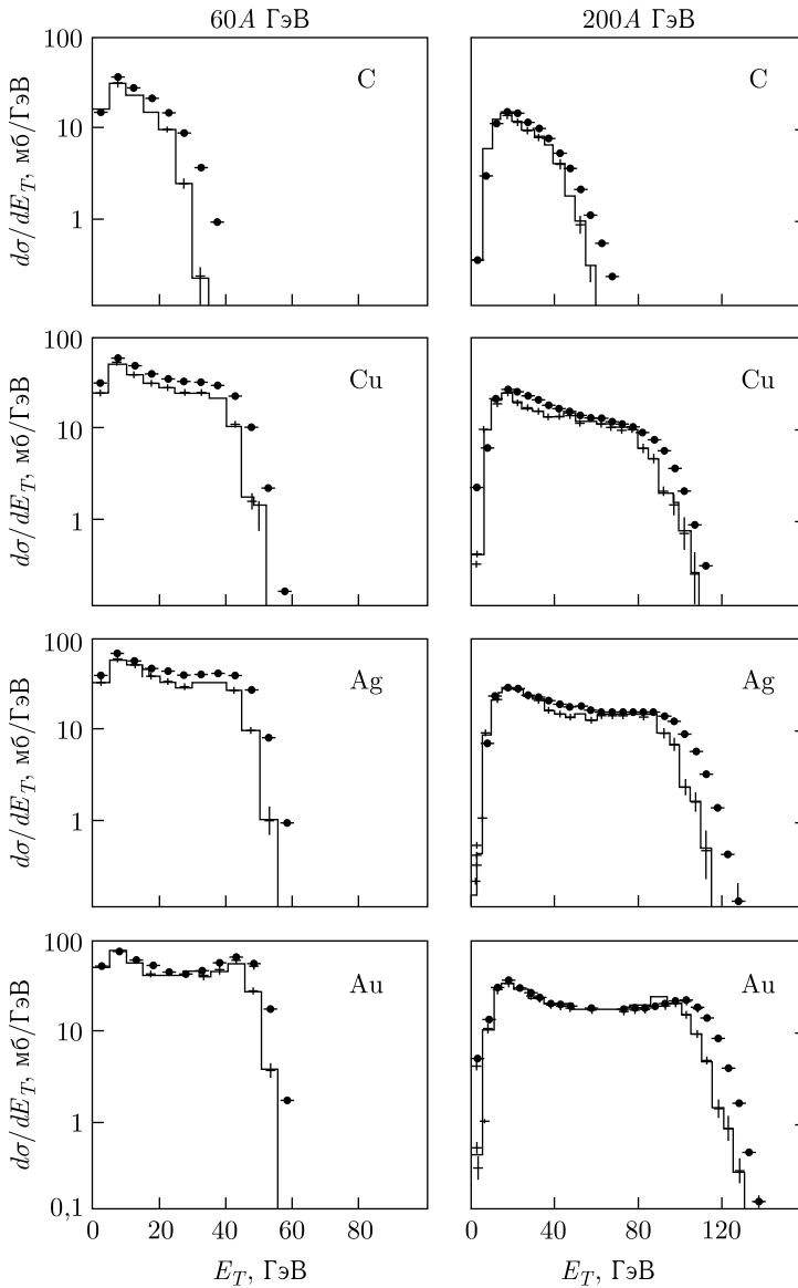
Рис. 5.7. Распределение по энергии в центральном калориметре для ядер C, Cu, Ag, Au при начальных энергиях 60 и 200А ГэВ. Гистограммы — расчет по модели FRITIOF [8]
