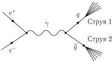
Рис. 1.5. Диаграмма двухструйного события
