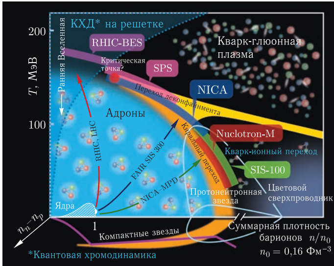
Рис. 4.3. Детальный вид фазовой диаграммы ядерной материи. Указаны области, доступные для исследований в различных ускорительных центрах мира. По вертикальной оси — температура T , по горизонтальной — барионная плотность ядерной материи, нормированная на обычную плотность n/n_0
