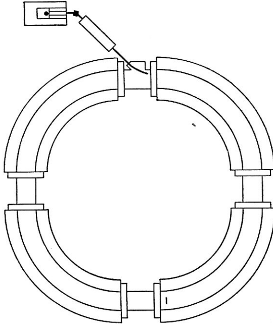
Рис. 4.2. Бэватрон Калифорнийского университета порождает антипротоны, ускоряя протоны до энергии 6,2 миллиарда электрон-вольт (6,2 Бэв). На схеме изображены четыре магнитных сегмента, внутри которых ускоряются протоны. Радиус каждого сегмента равен 15 м. Протоны вводятся в эту установку двумя ускорителями, расположенными наверху. Медная мишень, в которой рождаются антипротоны, обозначена вертикальной чертой справа внизу.
