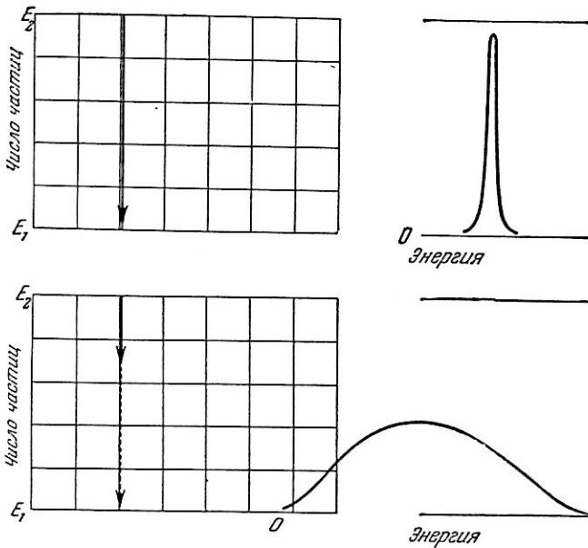
Рис. 3.4. Альфа- и бета-распады сопровождаются переходом ядра на другой энергетический уровень.
