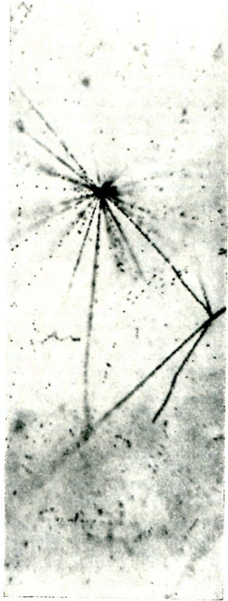
Рис. 6.6. Мезонная звезда, вызванная разрушением атома первичной частицей космического излучения.
