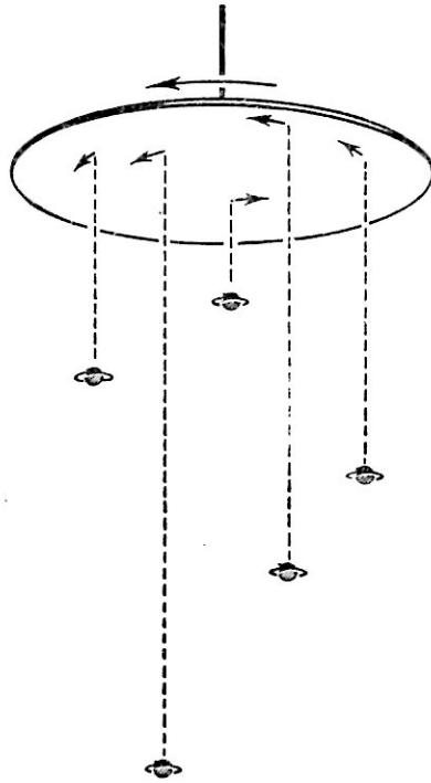
Рис. 7.8. Направление винта по крайней мере принципиально может быть определено с помощью алюминиевого диска, который может вращаться вокруг вертикальной оси. Нижняя сторона диска покрыта слоем кобальта-60. Электроны, испускаемые вниз, имеют преимущественно одно вращение (спин) и передают противоположное вращение диску. Испущенные вверх электроны поглощаются алюминием. Таким образом, диск все время вращается в указанном на рисунке направлении. Эта схема предложена Захарясом из Массачусетского технологического института.
