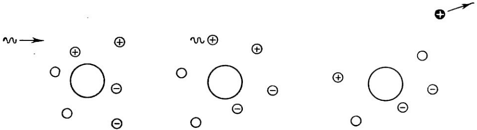
Рис. 2.3. «Виртуальный» пион материализуется, если системе сообщается энергия, превосходящая 135 Мэв. На рисунке гамма-квант большой энергии (волнистая линия) входит в мезонное облако и ударяет виртуальный положительный пион (светлый кружок). Энергия гамма-кванта поглощается, а виртуальный пион превращается в реальный (темный кружок). Теперь он может покинуть нуклон.
