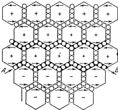
Рис. 8.1. Механическая модель электромагнитного поля, опубликованная в «Избранных трудах» Максвелла.
