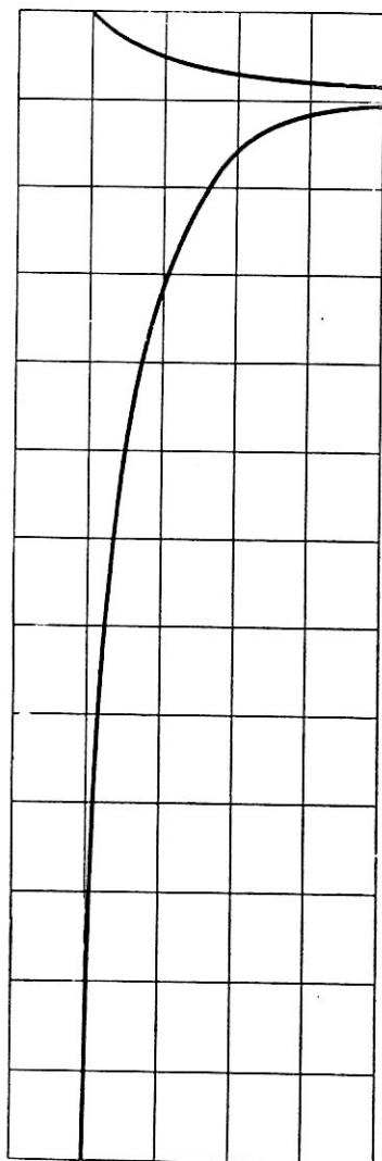
Рис. 2.6. Напряженности поля в случае электромагнитных и ядерных сил.
