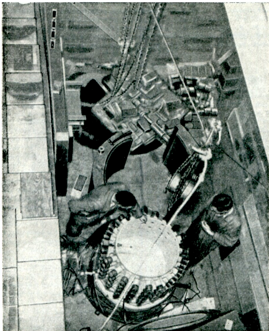
Рис. 3.7. Сцинтиляционный счетчик, использованный Райнесом, Кованом и их коллегами в попытке «поймать» нейтрино.
