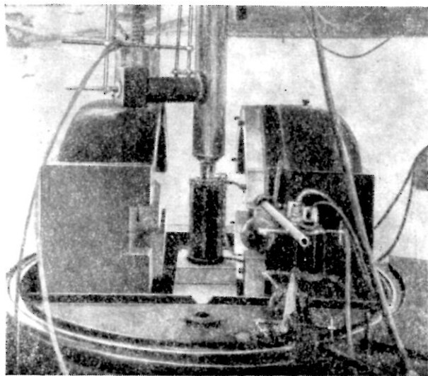
Рис. 7.6. Прибор Ву — Эмлера регистрирует электроны, испускаемые ориентированными ядрами кобальта. Черный вертикальный цилиндр — катушка, которая дает ориентирующее поле. Горизонтальная труба — фотоумножитель
