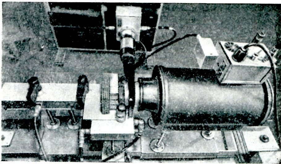
Рис. 6.3. Мезонная мишень.
