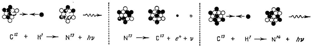
Рис. 3.2. Углеродный цикл — второй ядер
