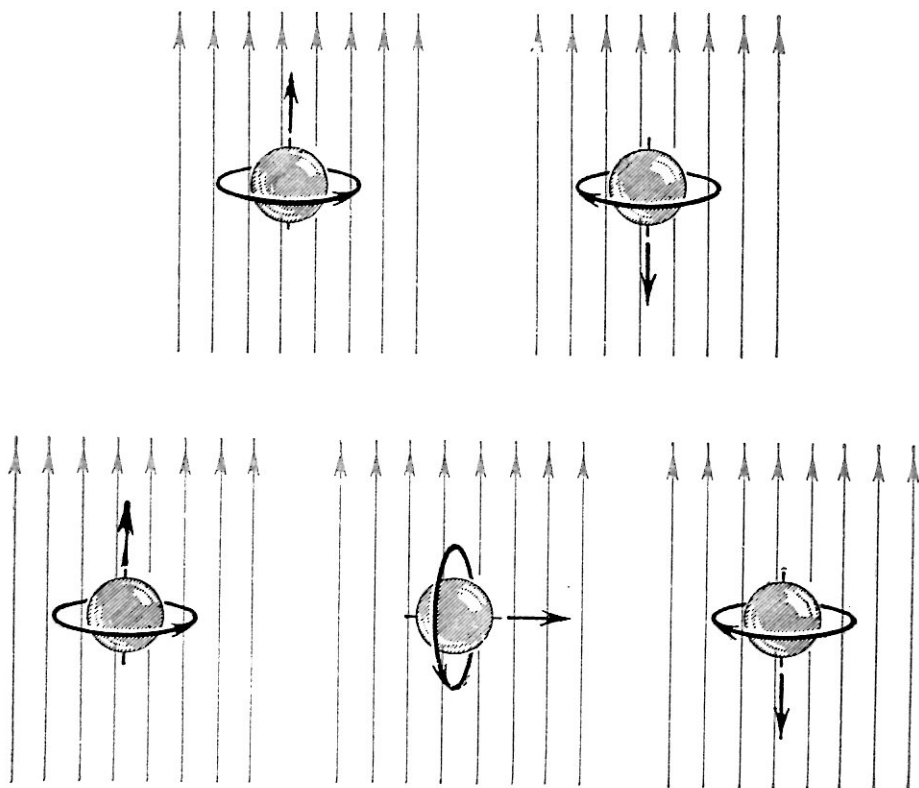
Рис. 1.1. Вращающаяся частица может принимать только некоторые фиксированные положения по отношению к внешнему магнитному полю (цветные стрелки). Частицы со спином 1/2 (вверху) могут располагать свои оси вдоль или против поля. Частицы со спином 1 (внизу) — вдоль, против и перпендикулярно к полю.
