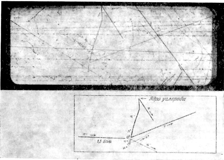
Рис. 7.3. Тета-частица ( \theta^0 ) распадается на два пи-мезона.
