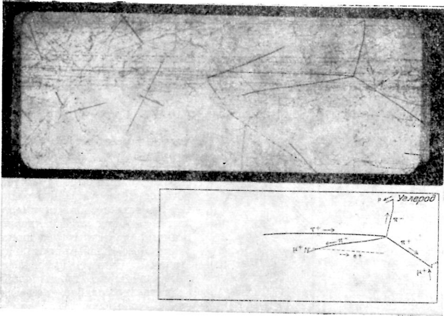
Рис. 7.2. Тау-частица ( \tau^+ ) распадается на три пи-мезона.
