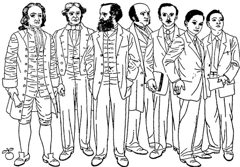
Рис. 8.3. Воображаемая компания физиков
