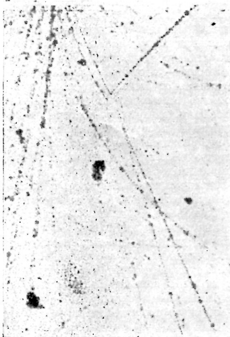
Рис. 1.5. Отрицательная кси-частица распадается на нейтральную лямбда-частицу и отрицательный пион. Лямбда-частица распадается затем на протон и второй отрицательный пион.
