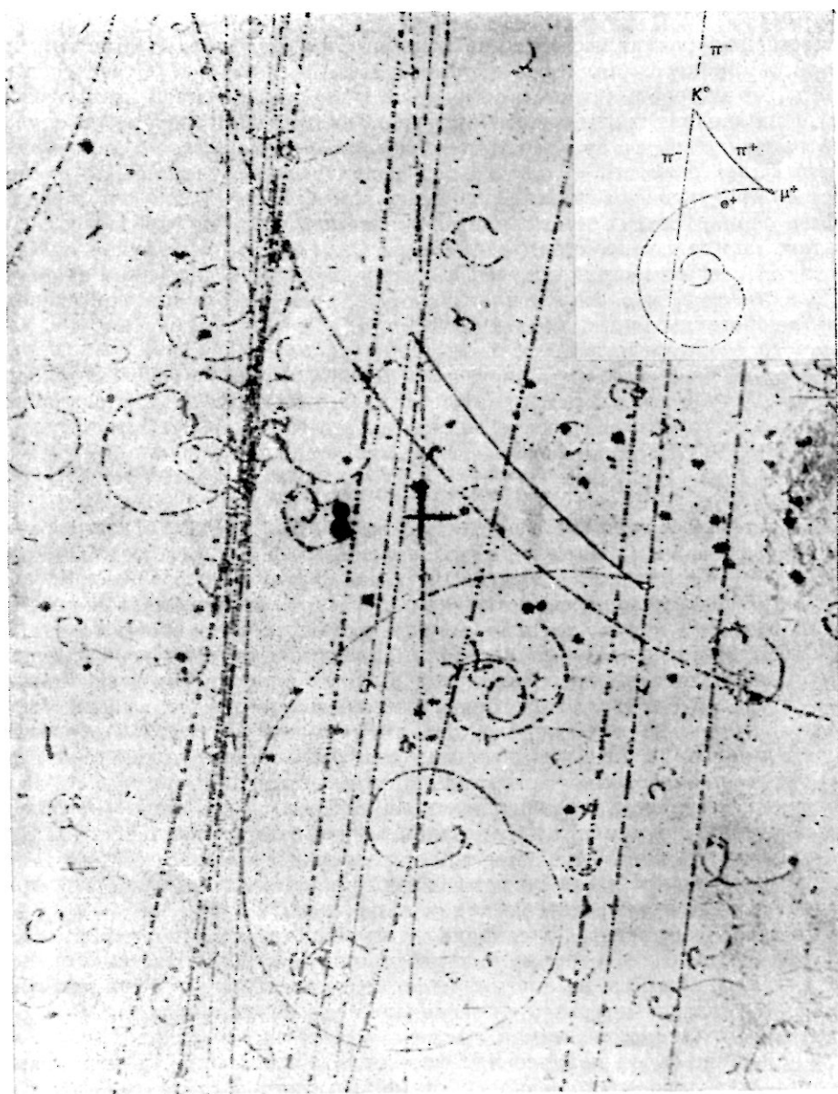
Рис. 1.3. Нейтральная K -частица, образовавшаяся при столкновении отрицательного пиона и протона, распадается на пару противоположно заряженных пионов, как это показано на схеме справа вверху.
