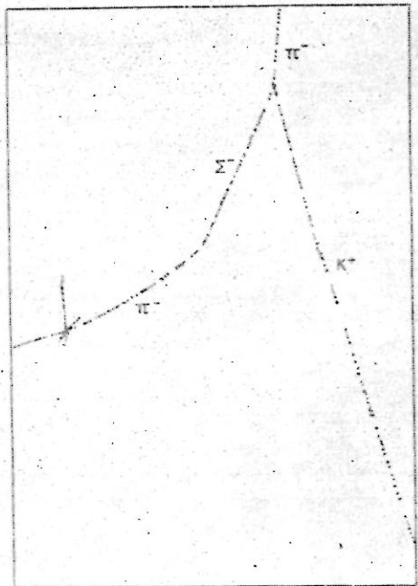
Рис. 1.4. Сигма и K -частицы образовались одновременно, когда пион ударил по протону в пузырьковой камере. Сигма-частица распалась на пион и невидимый нейтрон. Пион затем попал в ядро углерода и образовал «звезду» (см. схему справа).
