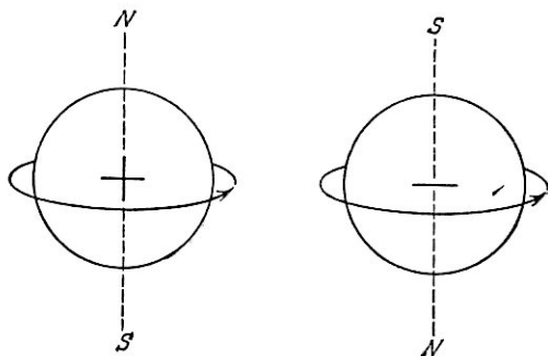
Рис. 4.1. Протон (слева) может грубо наглядно рассматриваться как вращающаяся сфера весом в 1,6724 \cdot 10^{-24} г. Он имеет положительный электрический заряд, и, в результате вращения, северный и южный магнитные полюса. Антипротон (справа) имеет тот же самый спин и массу. Он обладает электрическим зарядом такой же величины, знак которого, однако, противоположен. Поэтому его северный и южный магнитные полюса (по отношению к полюсам протона) переставлены.
