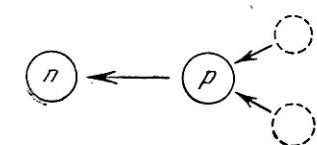
Рис. 1.2. Схема основных процессов.
