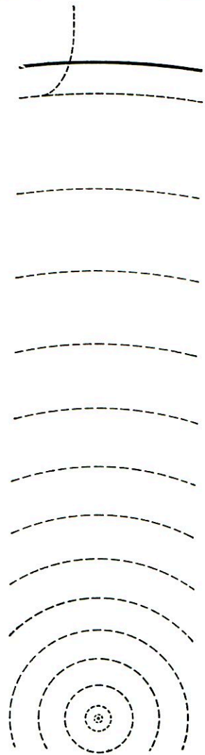
Рис. 6.4. Приближенная картина мезонных орбит углерода и их относительных расстояний от ядра атома (внизу).
