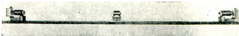
Рис. 5.2. Аннигиляция пара-позитрония обнаруживается двумя сцинтилляционными счетчиками (слева и справа).
