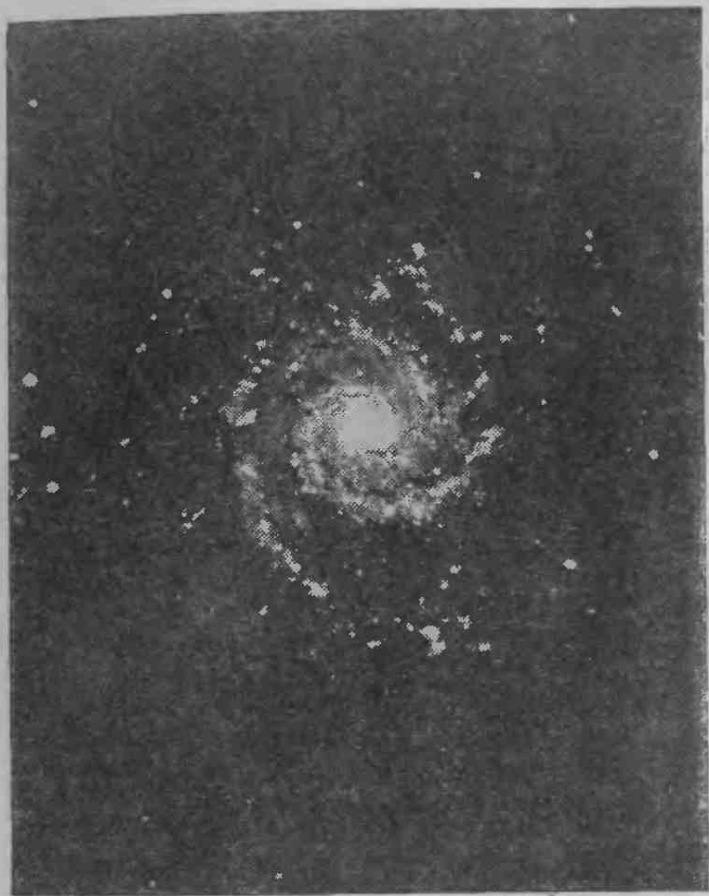
Рис. 8. Спиральная галактика
