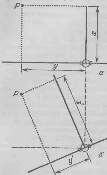
Рис. 26. a — положение точки P относительно меня характеризуется двумя числами x и y ; число x показывает, насколько далеко вперед ушла от меня точка P , а число y — насколько она смещена влево. б — положение той же самой точки P характеризуется двумя другими числами, если я стою на прежнем месте, но повернулся в сторону
